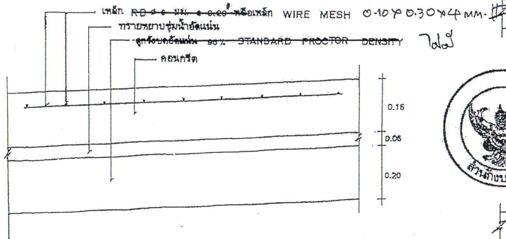
รายละเอียดคอนกรีตเสริมเหล็ก not to scale
