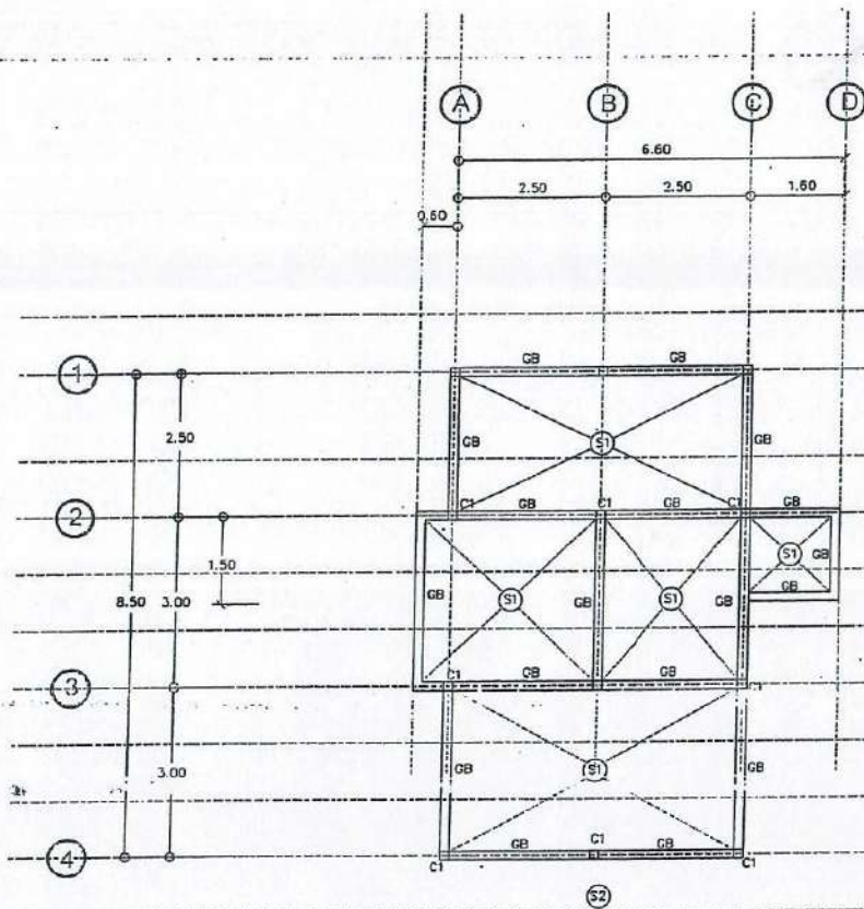
แปลนคาน , เสา , พื้น scale 1 : 100
