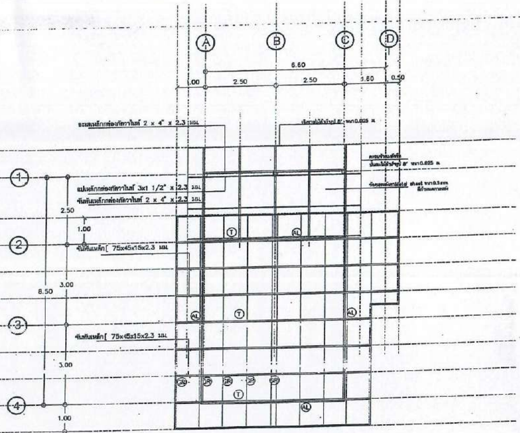
แปลนโครงหลังคา scale 1 : 100
